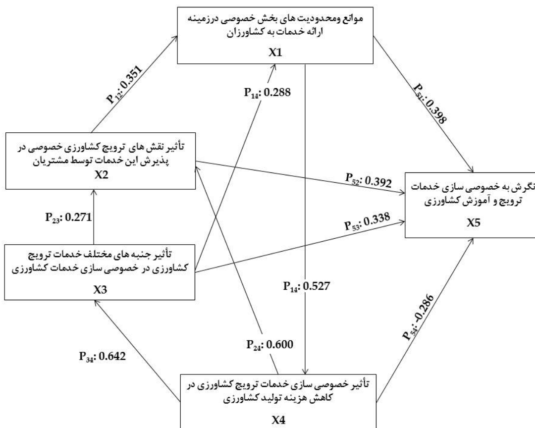
نگاره ۶- نمودار تفکیک شده از مدل علی نهایی تحلیل مسیر
